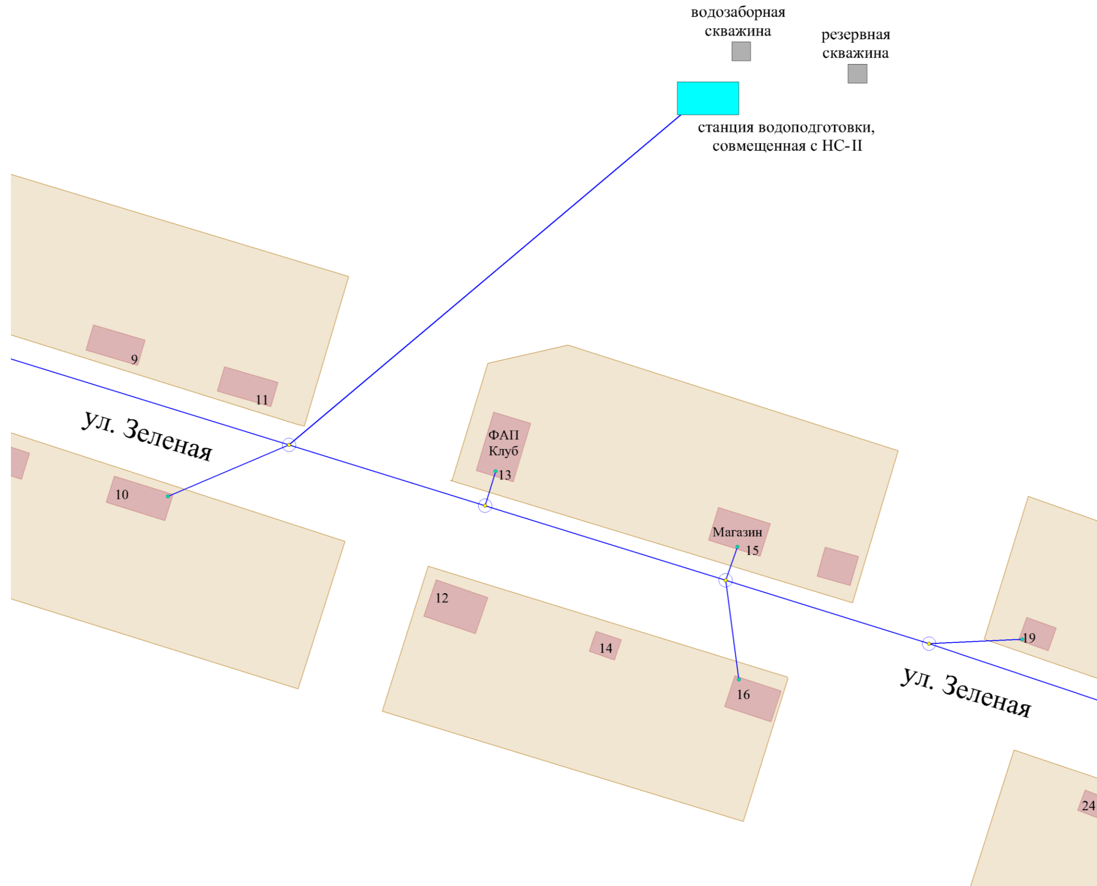
Рисунок 6.4 – Схема планируемого размещения объектов централизованной системы водоснабжения
