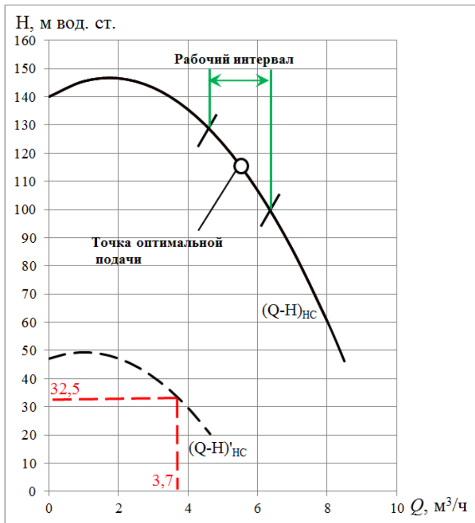
Рисунок 6.1 – Анализ характеристики насоса, установленного в водозаборной скважине (Q-H)_{НС} – характеристика насосной станции при одном работающем насосном агрегате при номинальной частоте двигателя; (Q-H)'_{НС} – характеристика насосной станции при одном работающем насосном агрегате при частоте двигателя сниженной на 42%.
